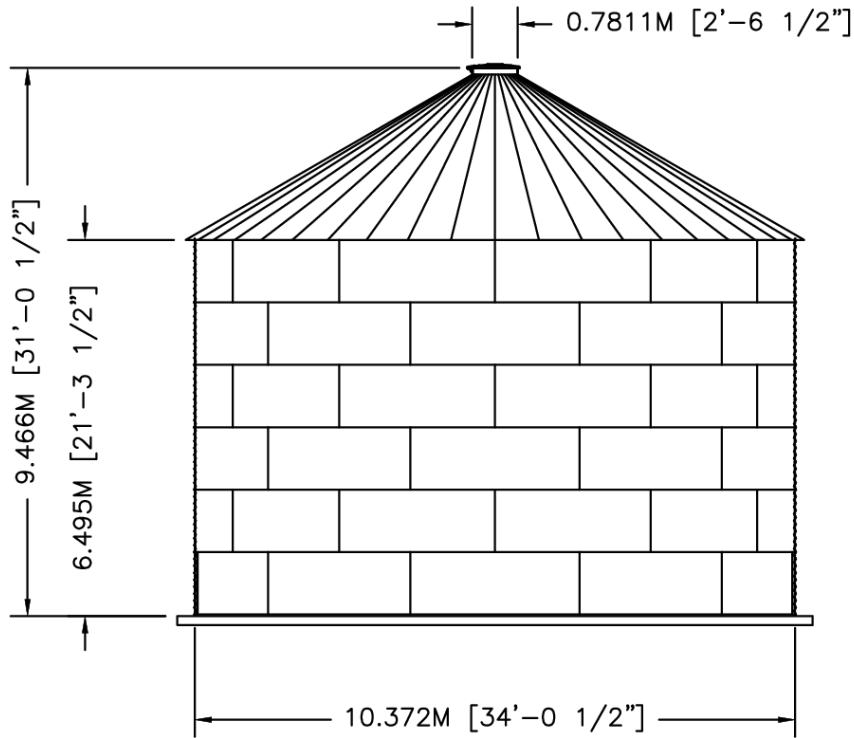
ELEVATION
